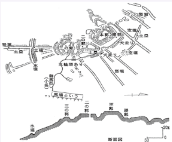
替佐城の図面
