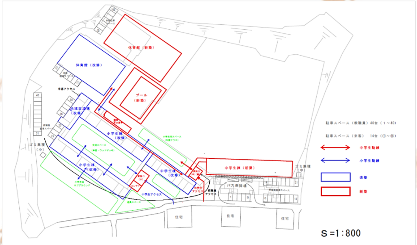
豊田地域小学校統合計画敷地配置図（案）
