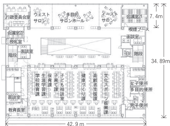
▲ 2階 (床面積 1,417.51㎡、天井高さ 2.7m)
