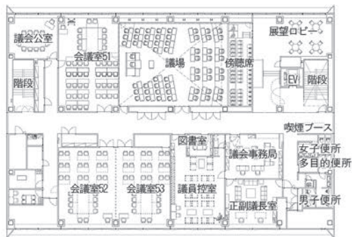
▲ 5階 (床面積 1,208.92㎡、天井高さ*2.7m) *議場部分は 5.8m
