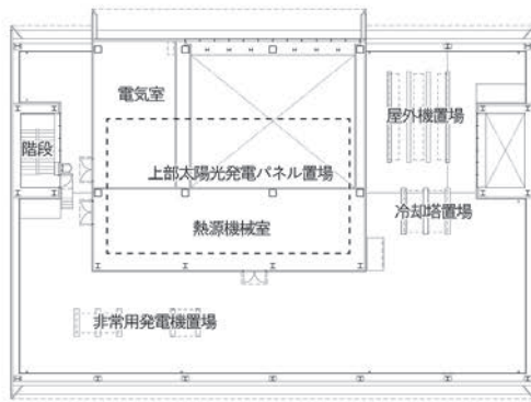
▲ 6階 (R階) (床面積 264.60㎡)
