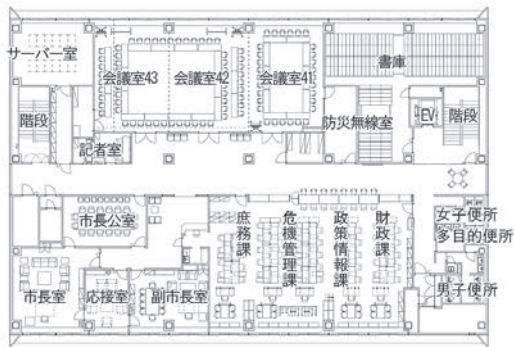
▲ 4階 (床面積 1,208.92㎡、天井高さ 2.7m)
