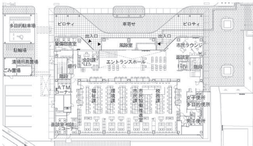
▲ 1階 (床面積 1,162.36㎡、天井高さ 3m)
