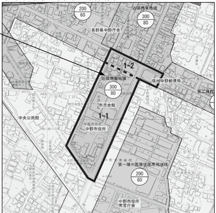
中野市用途地域変更 計画図
